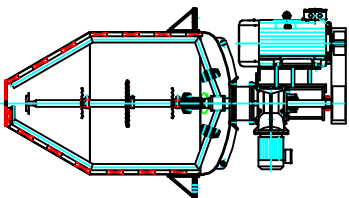
KONUSMISCHER MIT DISSOL VERANTRIEB
