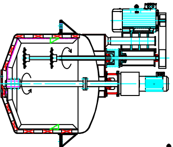
MISCHER MIT ANKERANTRIEB UND DISSOL VERANTRIEB VON OBEN
